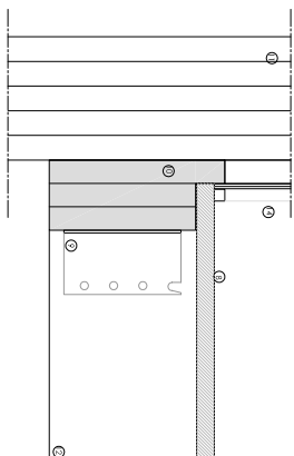
SECCIÓ - DETALL 2
